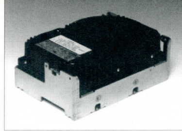
◀日立製5インチ・フルハイトの330MB SCSIドライブ「DK514C-38」
