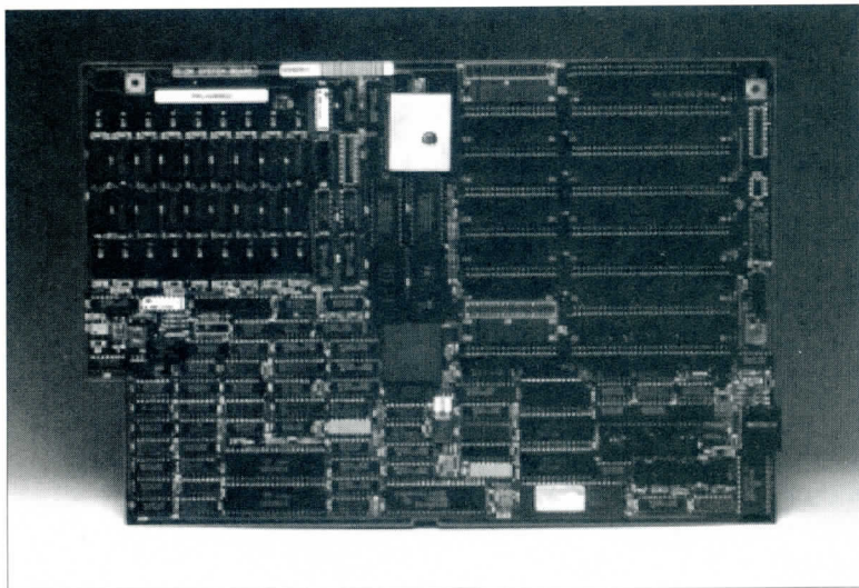
▲IBM PC/AT純正のマザーボード
