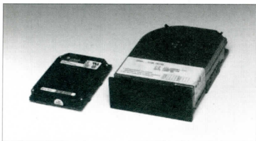
▲NEC製の40MB SCSI HDD「D3841」(右)と、CONNER社製2.5インチIDE HDD「CP-2024」
